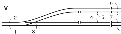
Weichenmotor mit Herzstückpolarisierung & Halteabschnitt & wählbarer Spannungsquelle
