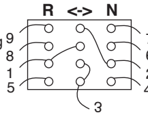
Weichenmotor mit Herzstückpolarisierung & Halteabschnitt & wählbarer Spannungsquelle
